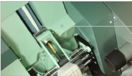
精梳機抗靜電導棉皮圈 VISBELT M-5E
